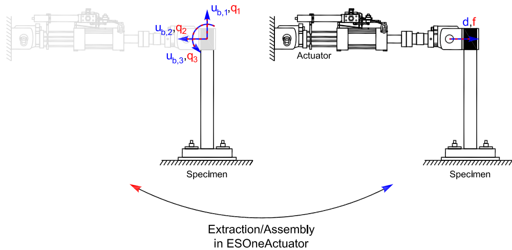
Fig. 3.23 One actuator experimental setup (ESOOneActuator).
